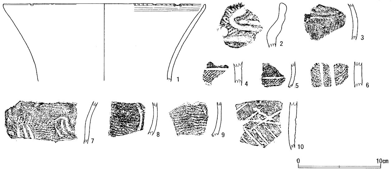
図8 2号竪穴住居址出土遺物 (1:3)
