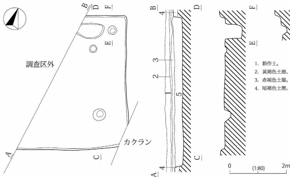
第7図 H4号住居址(1)
