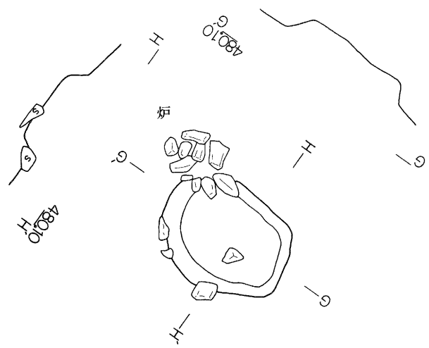
第5図 SB-02 実測図
