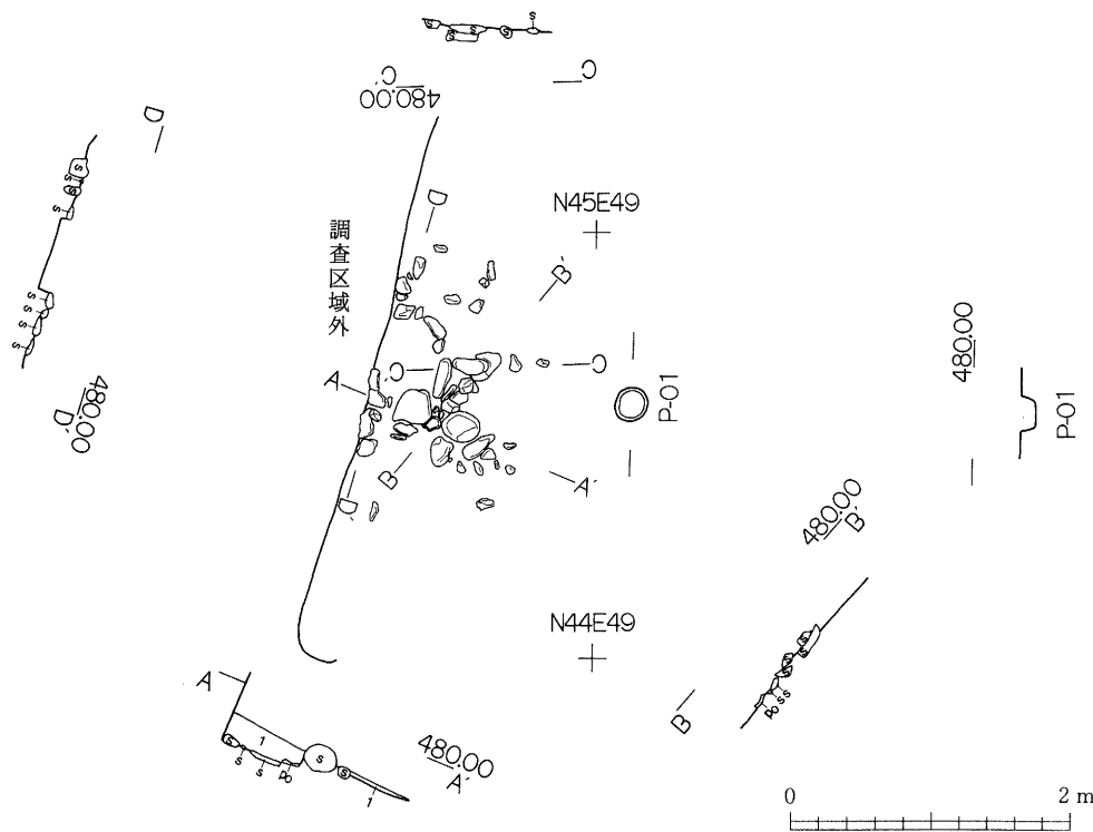
第9図 SX-01 実測図
