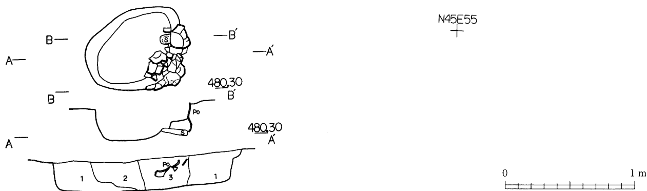
第10図 埋壙址実測図
