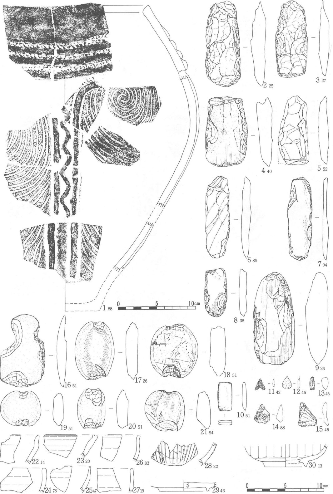
第4図 詳細分布調査グリッド出土主要遺物実測図2 (S=1/3)
