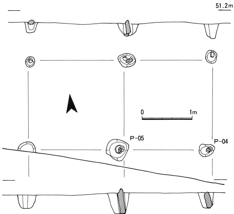
第9図 SB-02遺構平面図及び断面図 (S = 1 / 40)
