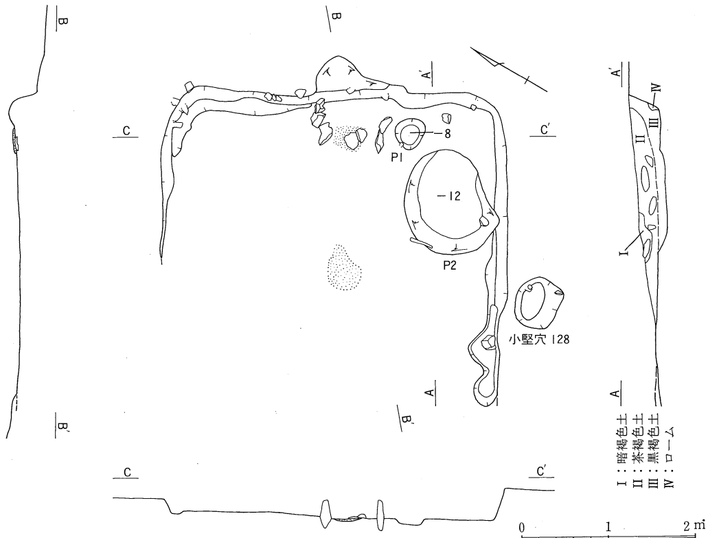
第11図 第1号住居址実測図 (1/60)
