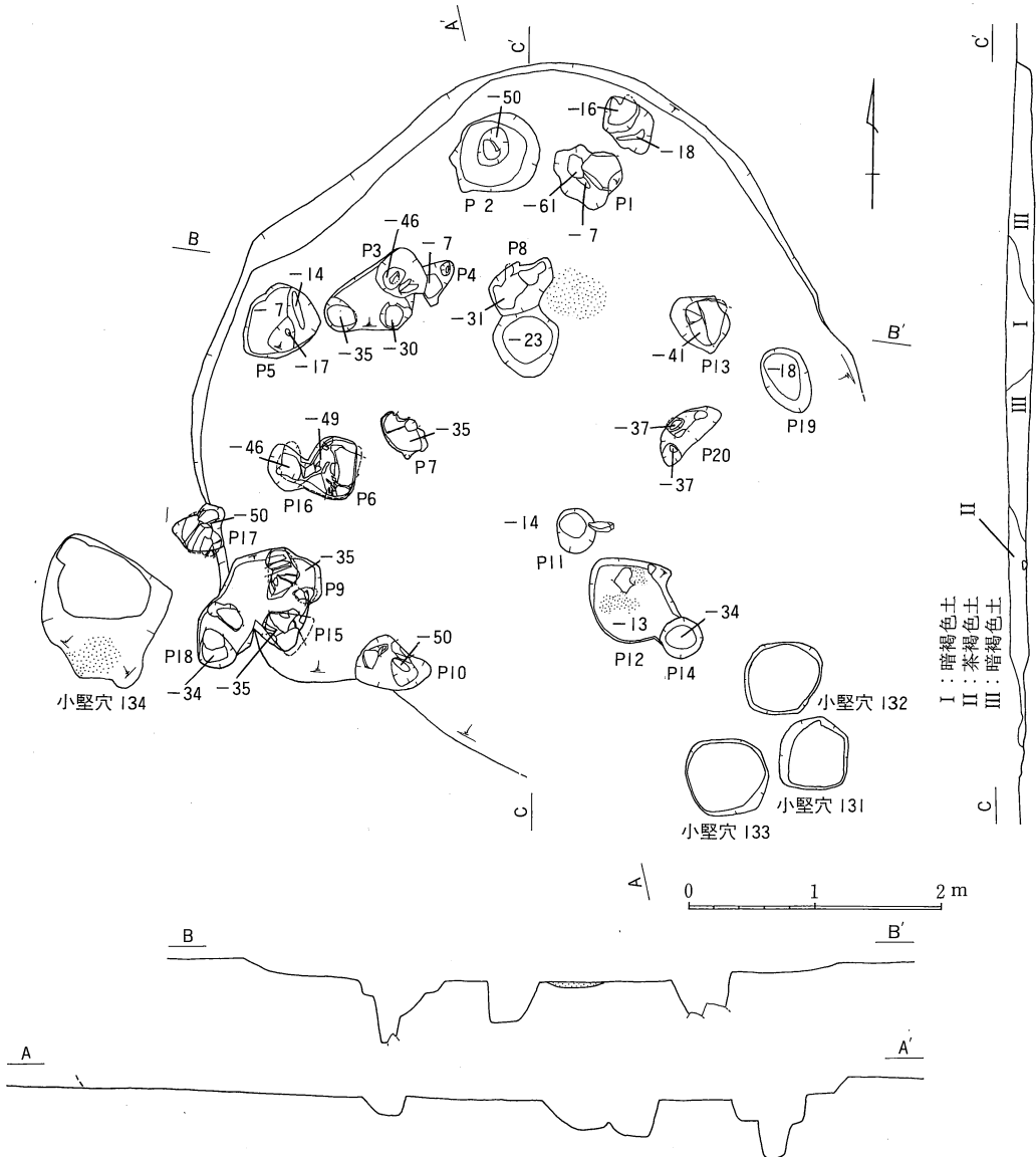
第4図 第5号住居址実測図 (1/60)
