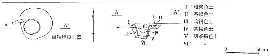
第10图 小堅穴・集石 I・单独埋設土器 I 実測図 (1/60・1/30)
