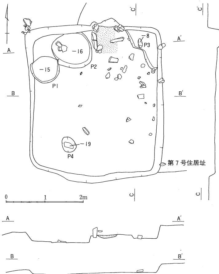
第13図 第3号住居址実測図 (1/60)
