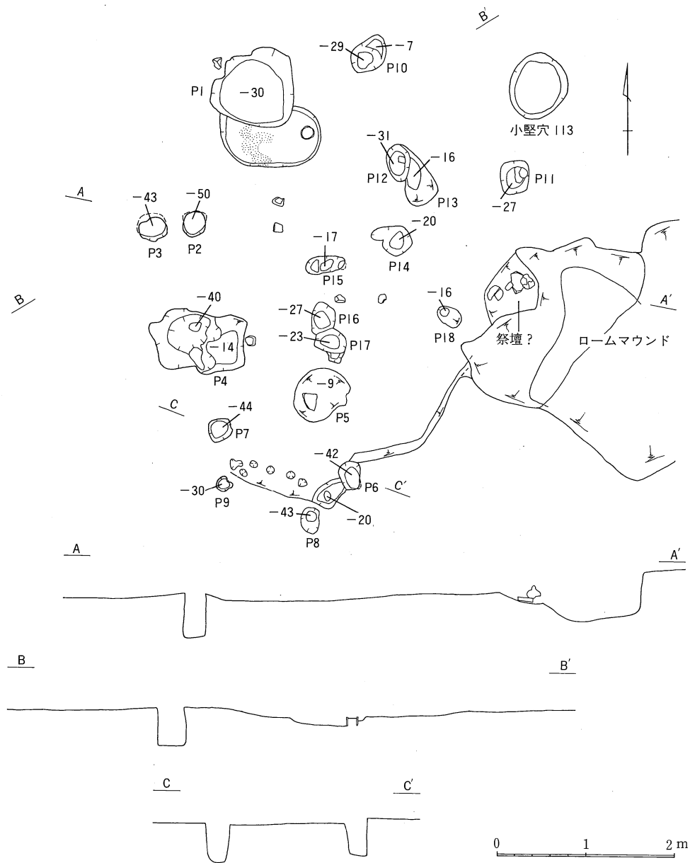
第5図 第6号住居址実測図 (1/60)
