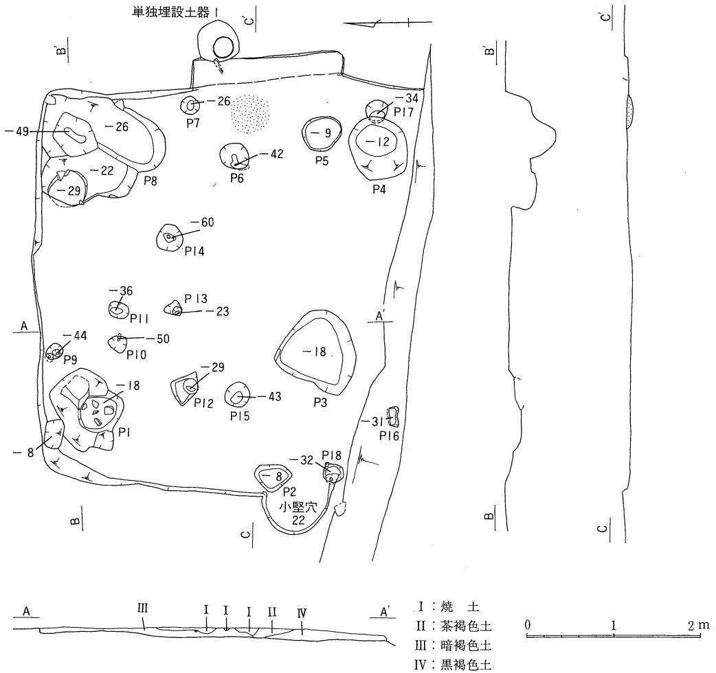
第12図 第2号住居址実測図 (1/60)
