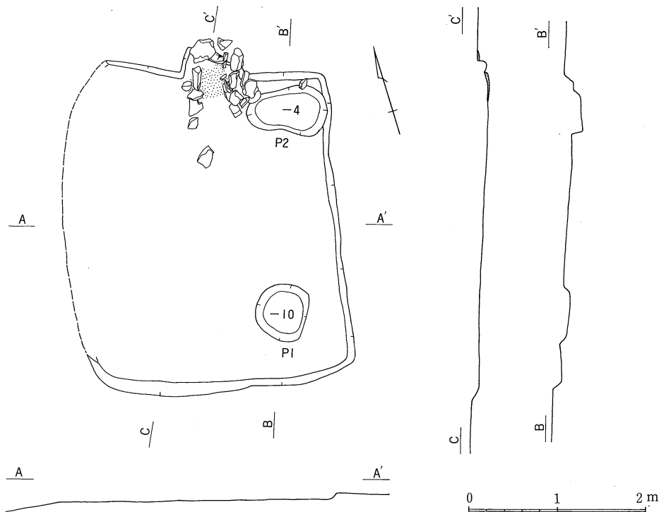
第15図 第4号住居址実測図 (1/60)
